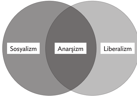
Şekil 5.1 Anarşizmin doğası
